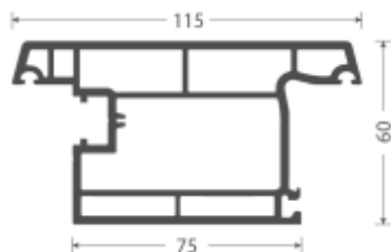
Casement Casement Door Sash AP-06
